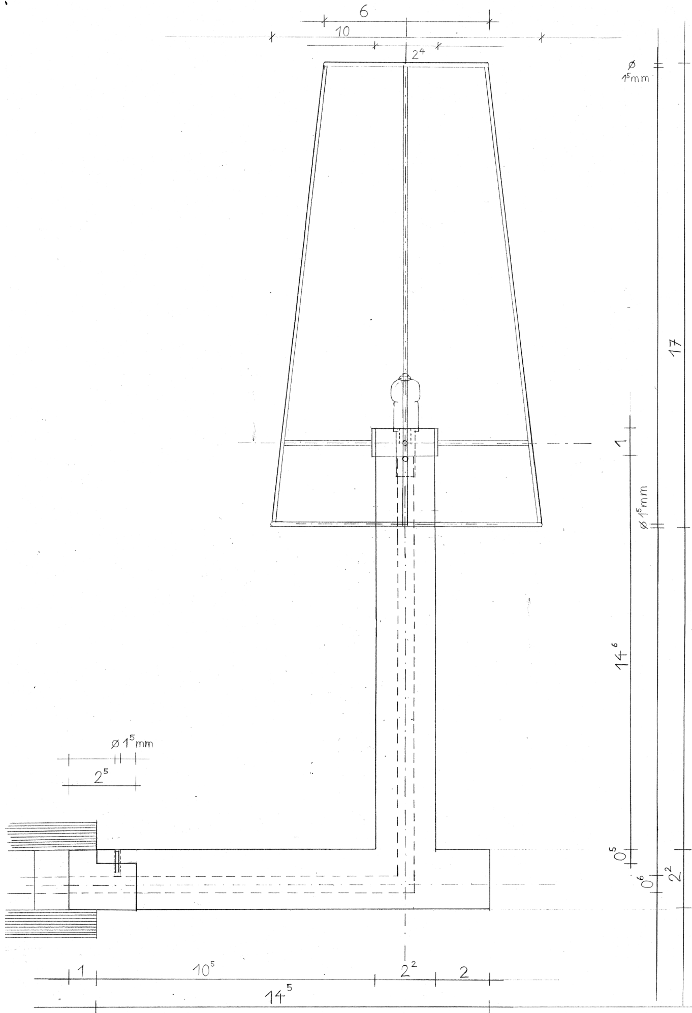
Schnitt M 1:1
